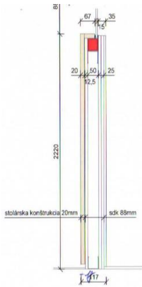
REZ 1-1 priečka v mieste dreveného obkladu
