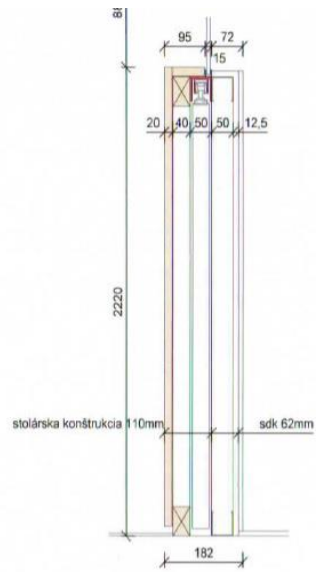
REZ 3-3 priečka v mieste dverného púzdra
