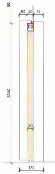
REZ 2-2 priečka v mieste drevených dverí
