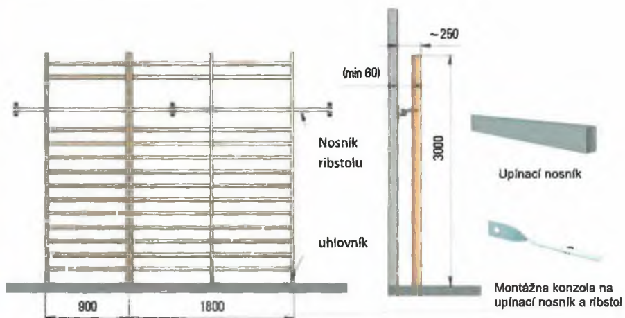
Ribstol montovaný na ocelovom nosníku
