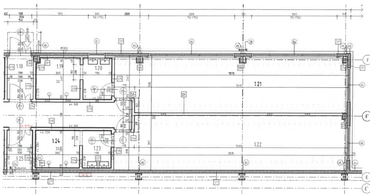
Pôdorys administratívneho prístavku DRS
