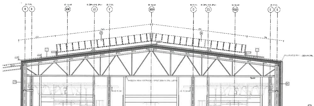
Tvar strešných väzníkov DRS
