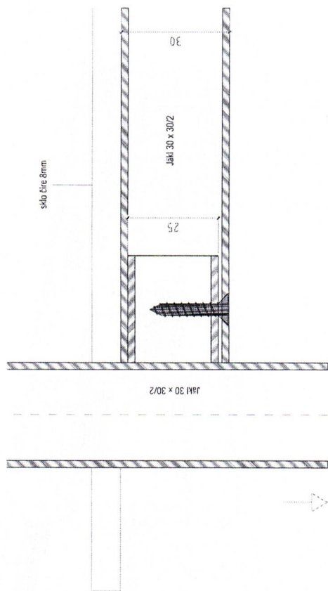
DETAIL D6 mierka 1:1
