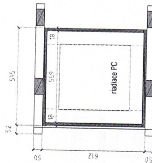
Pôdorys - Level L1 mierka 1:15
