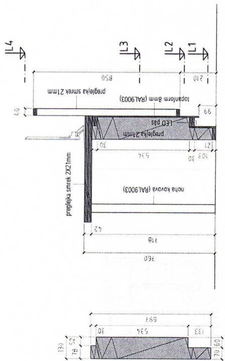
Rez A mierka 1:15
