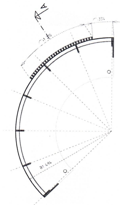
Pôdorys – Level L3 mierka 1:25
