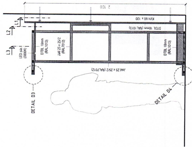
Vitrína - rez B-B mierka 1:20
