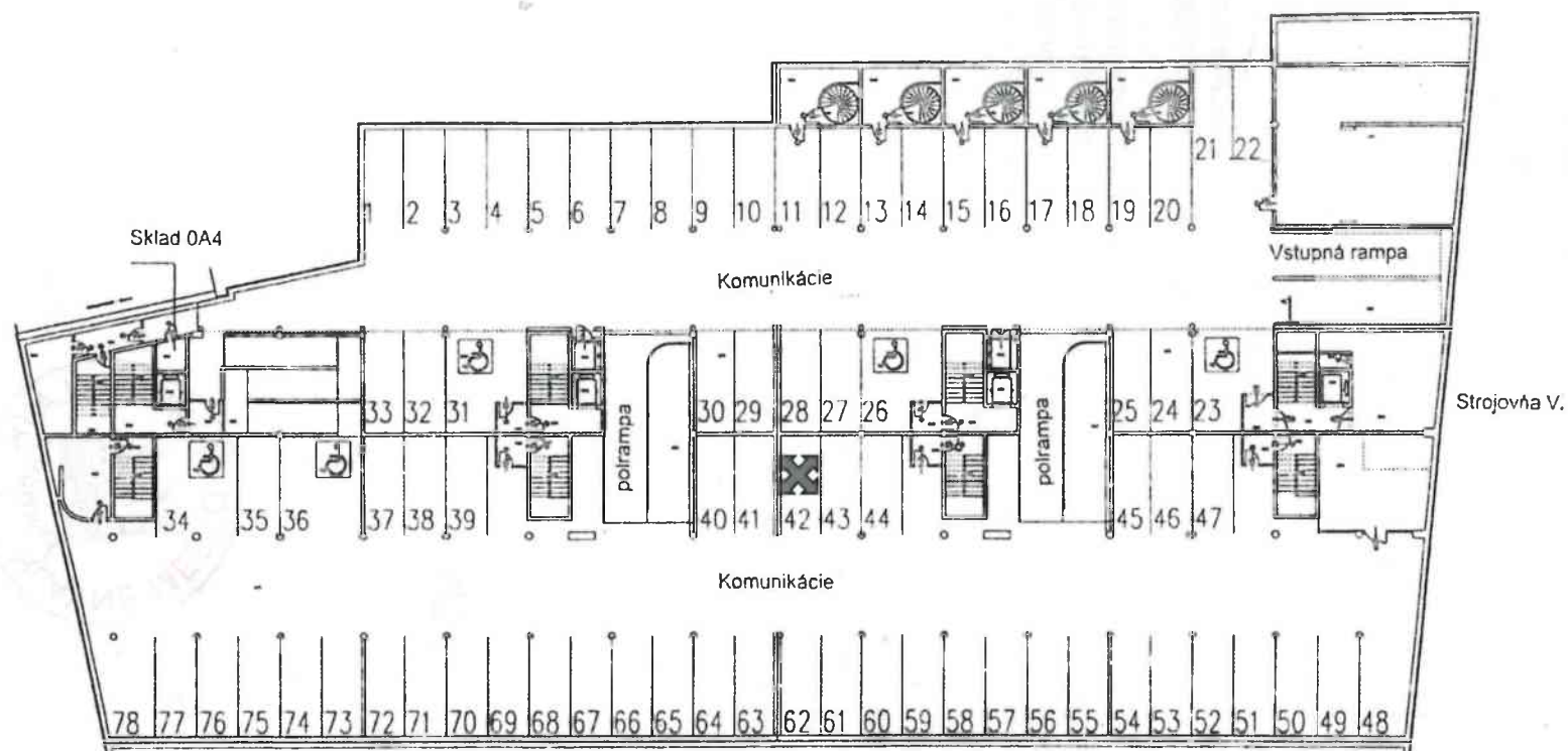
PÔDORYS 1. SUTÉRENU
