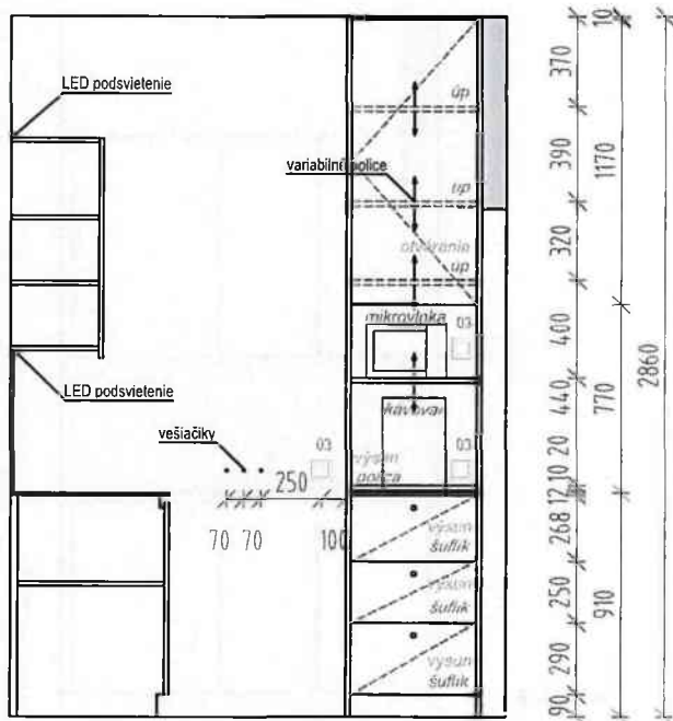
rezopohľad A-A'
