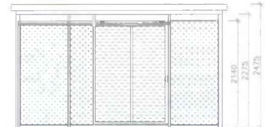
Pohľad čelný
