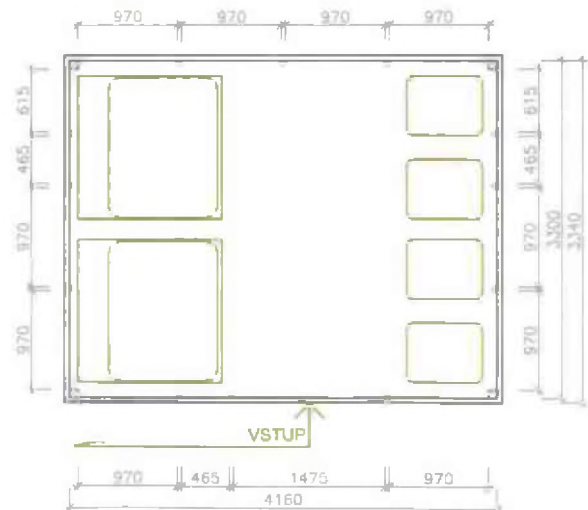
Pôdorys
