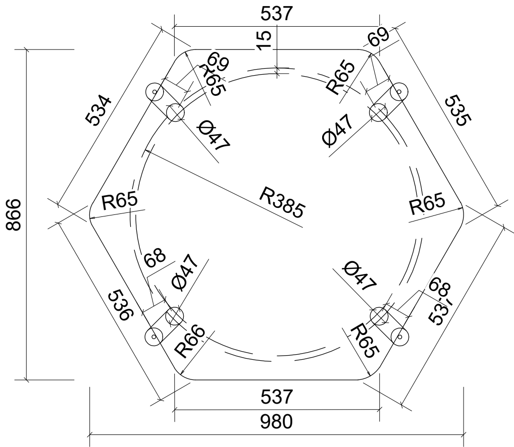
PÔDORYS 1:10
