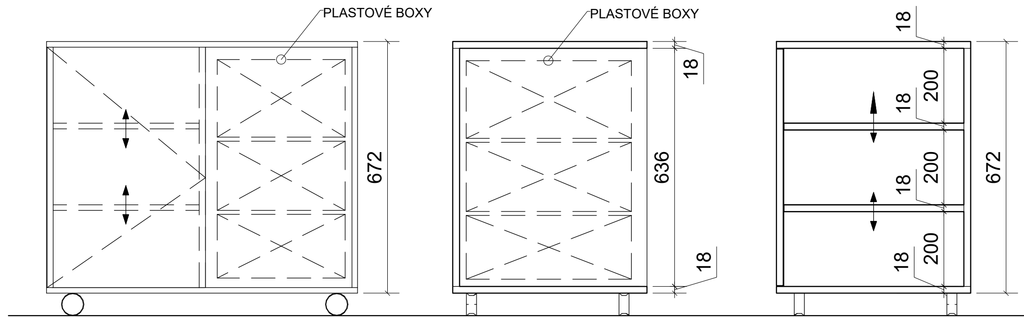
ČELNÝ POHĽAD 1:10
