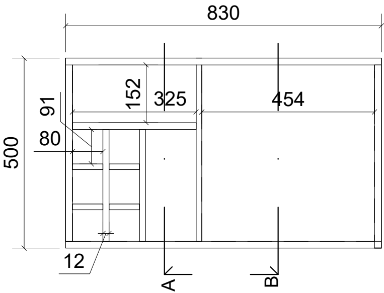
PÔDORYS 1:10
