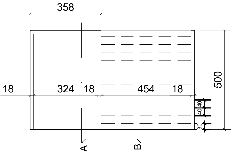
PÔDORYS 1:10
