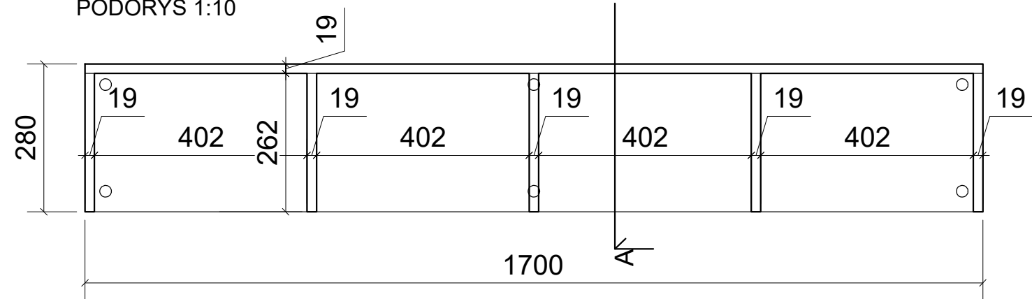
PÔDORYS 1:10
