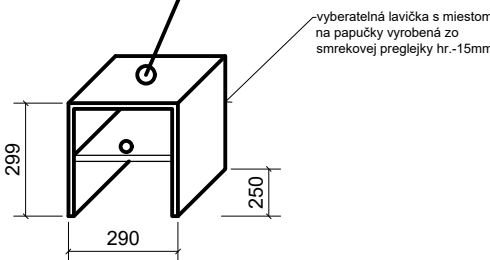
AXONOMETRIA
