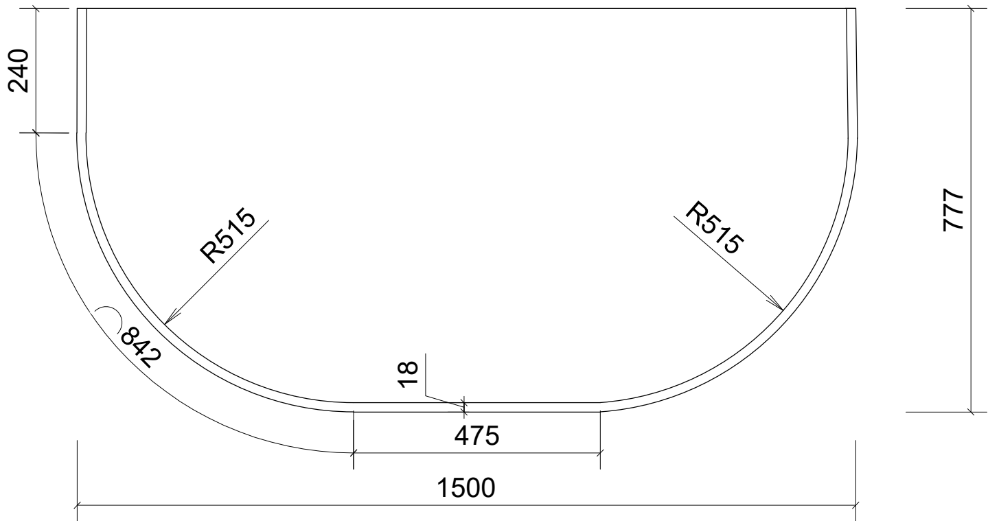
POHLAD 1:10
