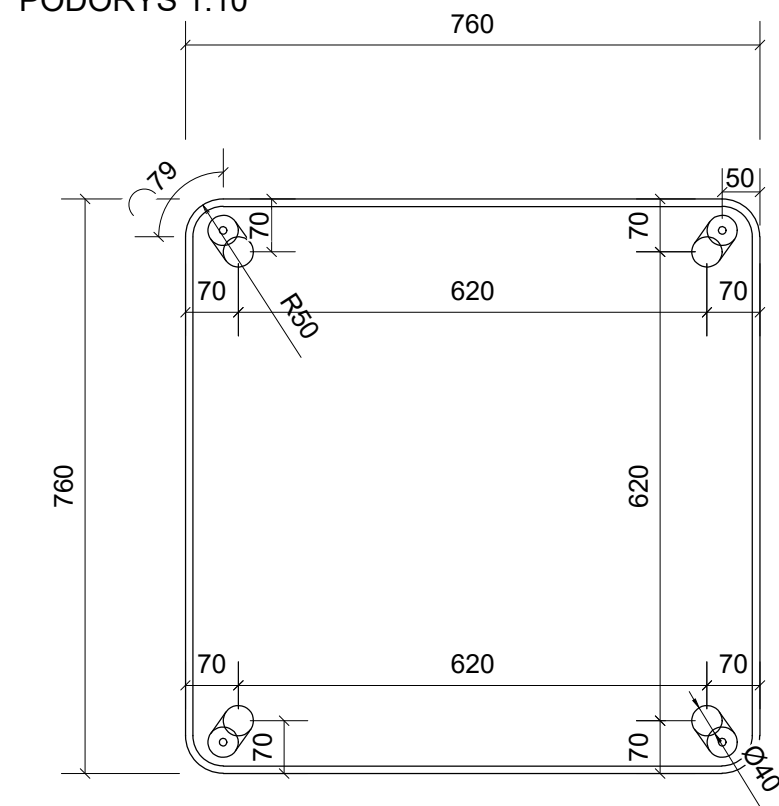
PÔDORYS 1:10
