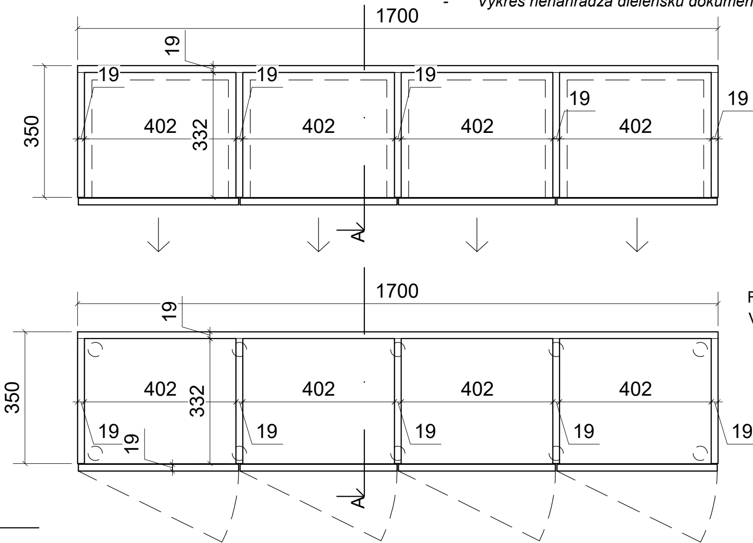
PÔDORYS 1:10
