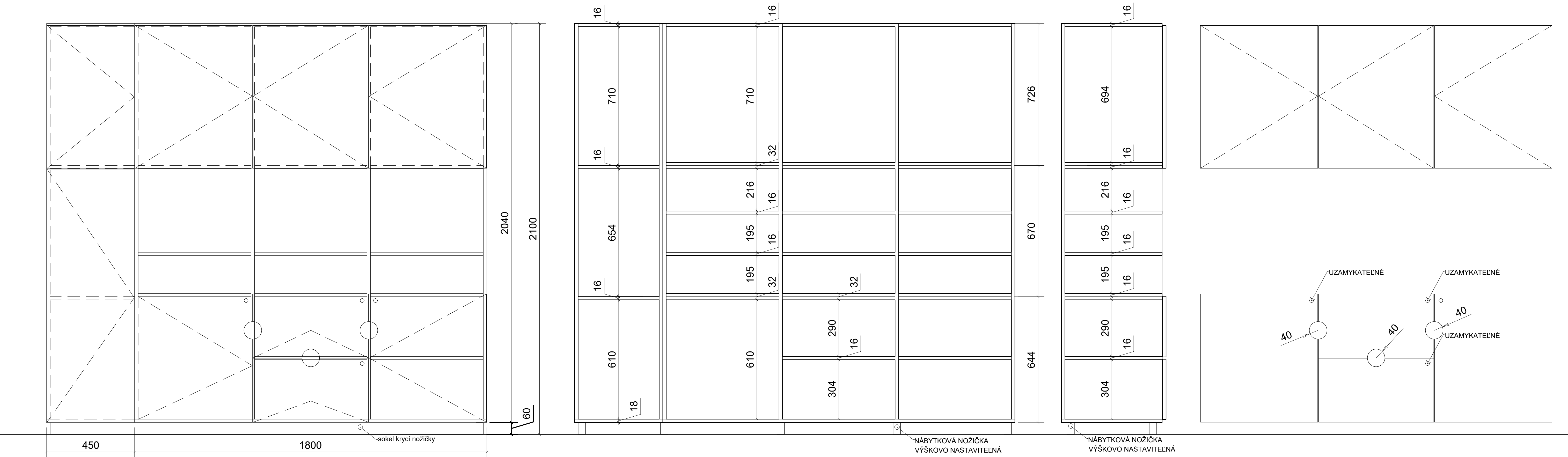
ČELNÝ POHĽAD NA DVIERKA 1:10
