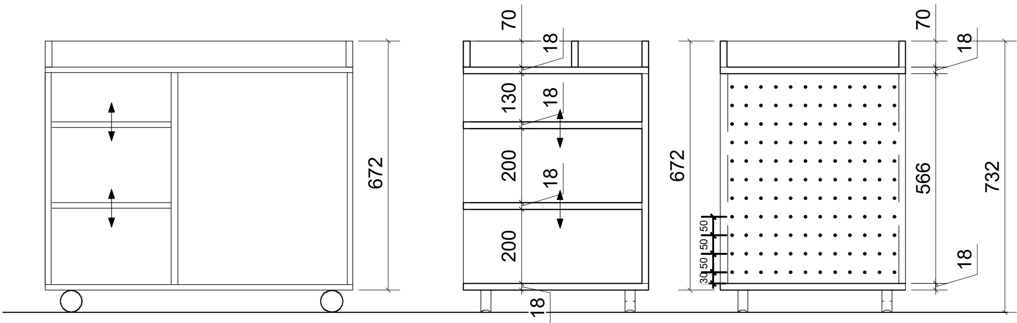
ČELNÝ POHĽAD 1:10
