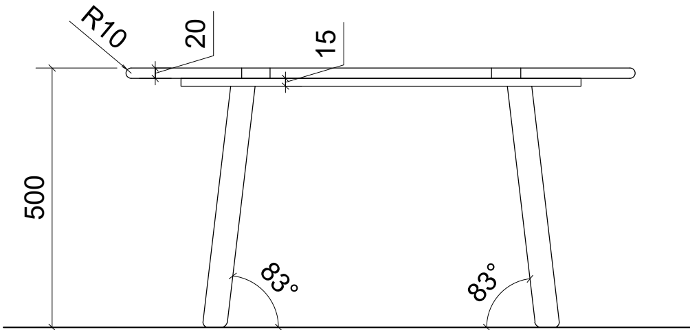
POHLAD 1:10
