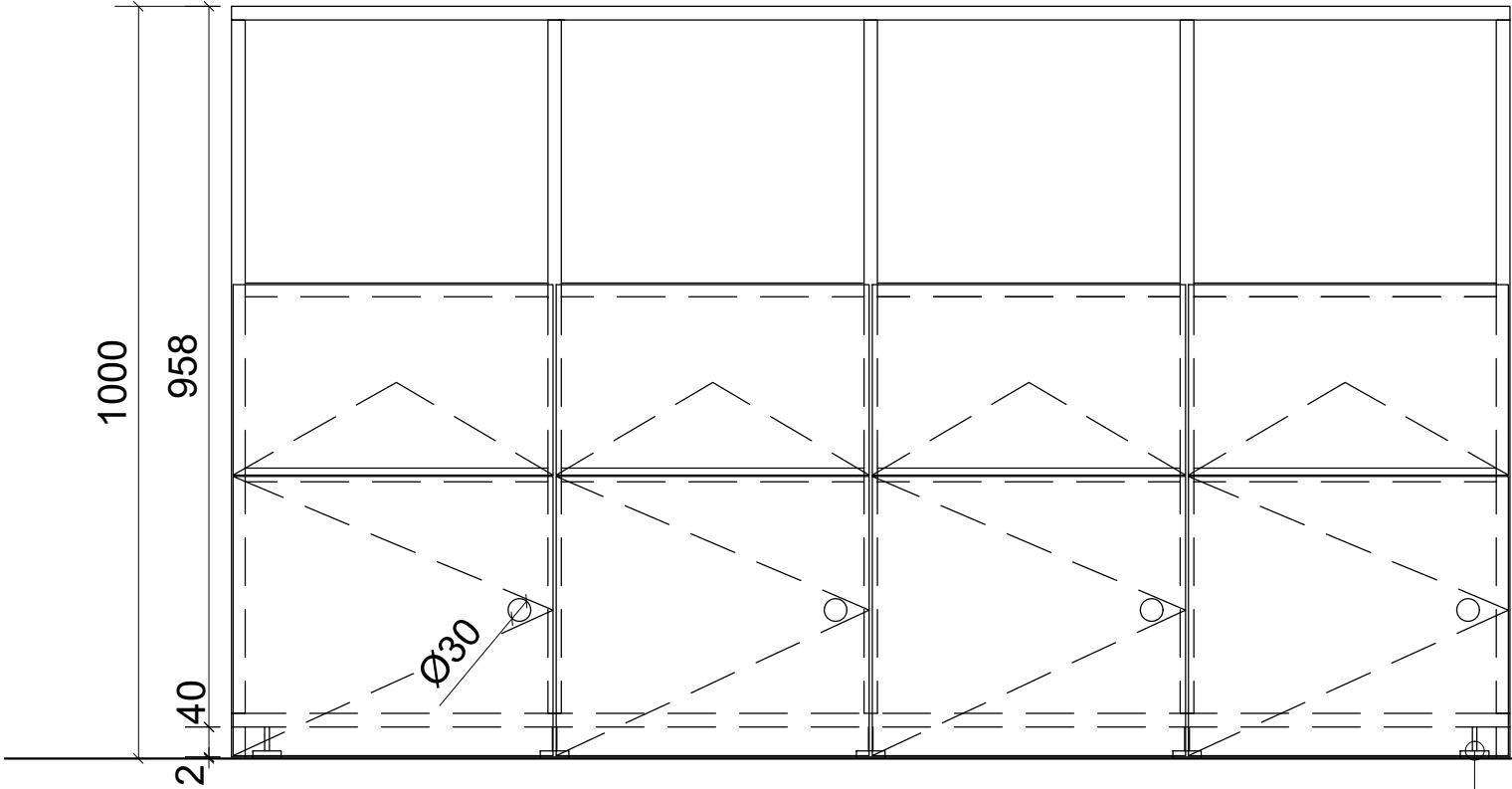
POHĽAD 1:10
