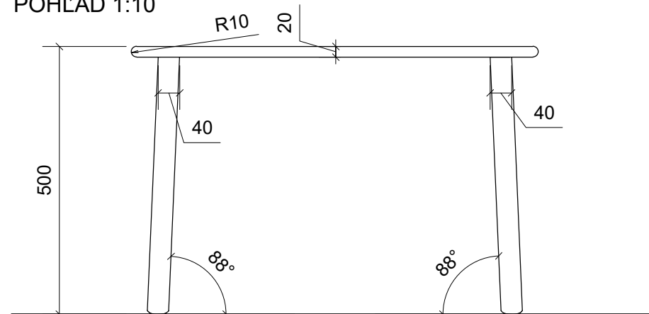
POHĽAD 1:10
