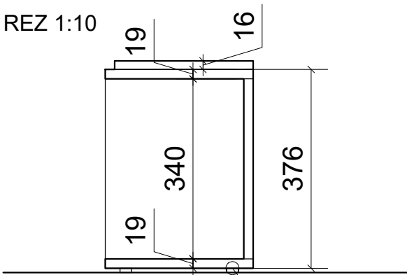
NÁBYTKOVÁ NOŽIČKA
