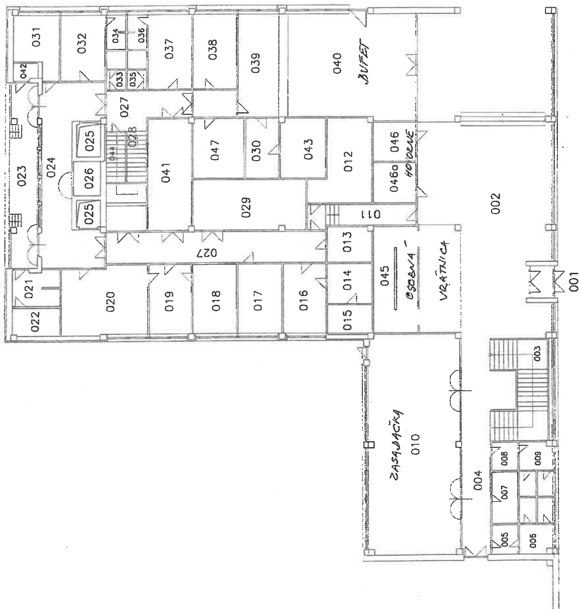
SMÚ BRATISLAVA - OBJEKT 'B' PÓDORYS pizemia
