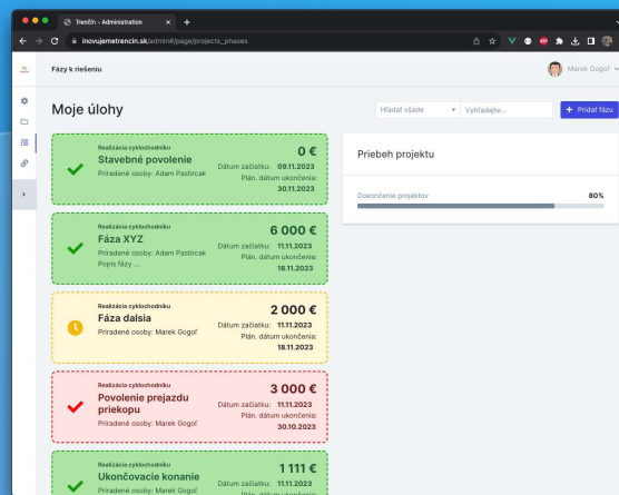
Úradnícke rozhranie
