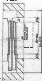
Detail dverí 1:20 Vstup 1. úrovn. (100/0)
