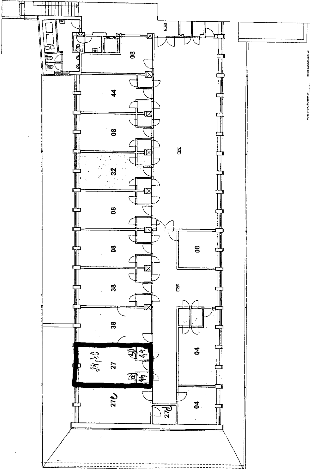
'AVILÓN "A" - PÓDORYS 1.POSCHODIA 1:120
