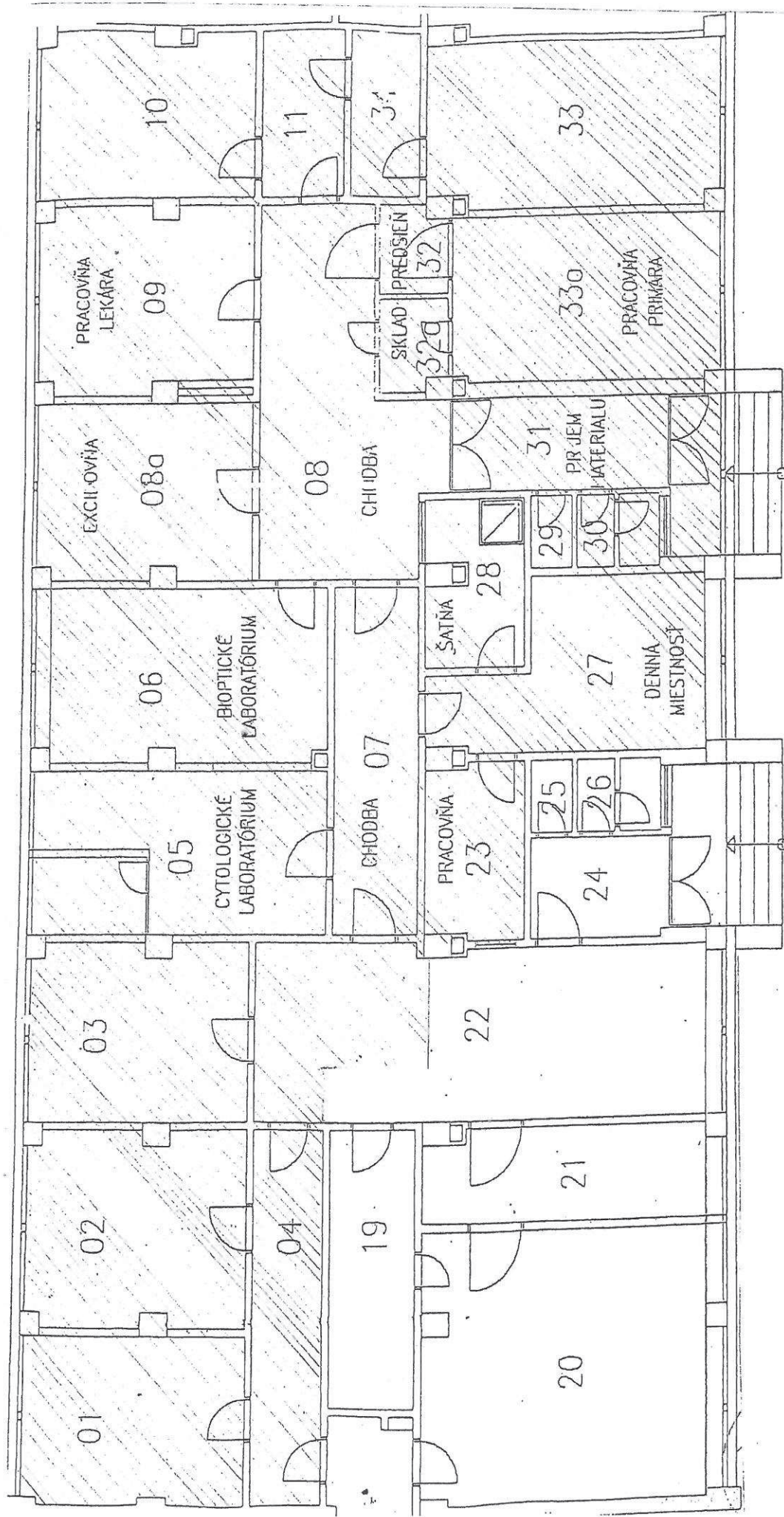
Pôdorys prízemia RÚVZ – časť A
