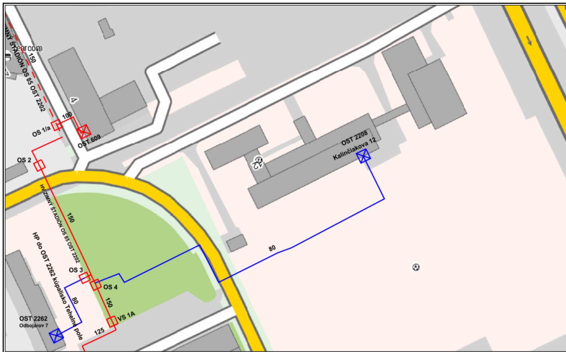
Príloha č. 1: Situácia horúcovodnej prípojky a OST
