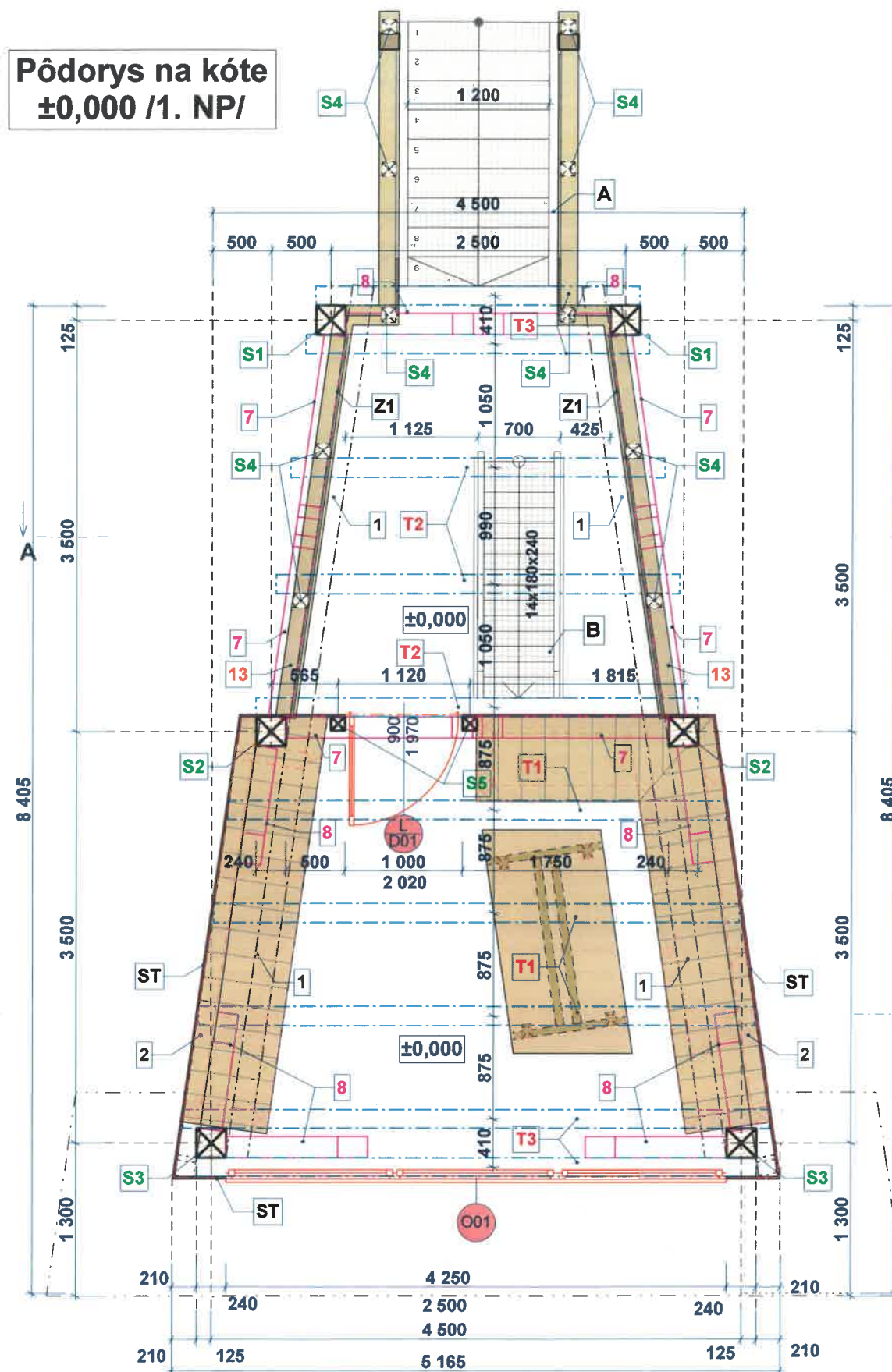
Pôdorys na kóte +3,360 /2. NP/
