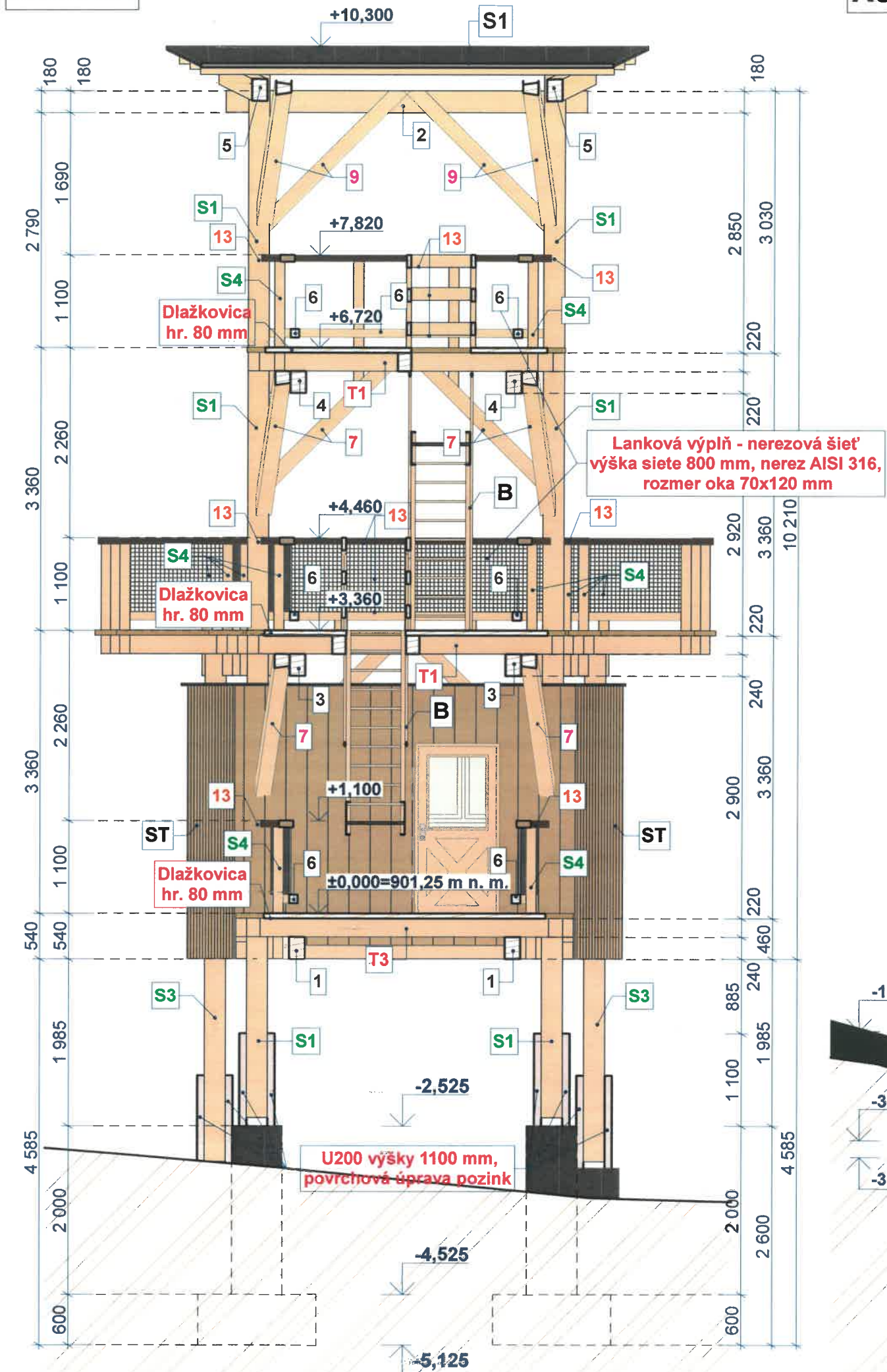
Rez A-A
