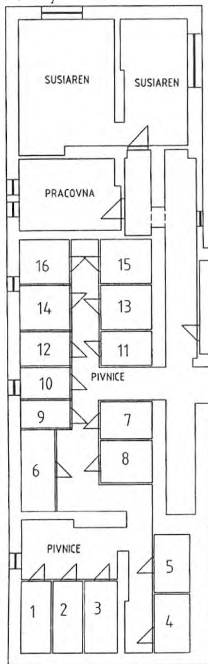
TRENCIANSKA 41, vlavo Podorys: Suterenu
