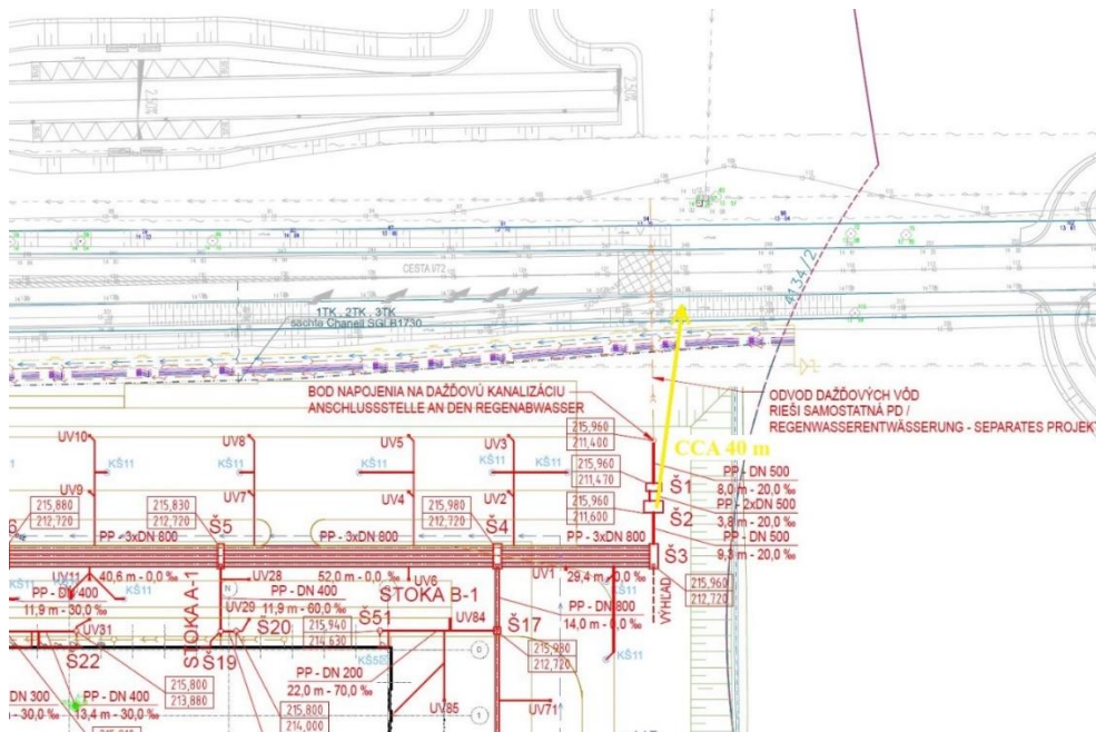
Obrázok č. 1 výkres a určenie vzdialenosti čerpania dažďovej vody zo šachty č.2 respektíve č.3 do cestného rigolu.
