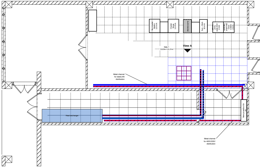
Obr. 4 : Položenie žľabov na kabeláže
