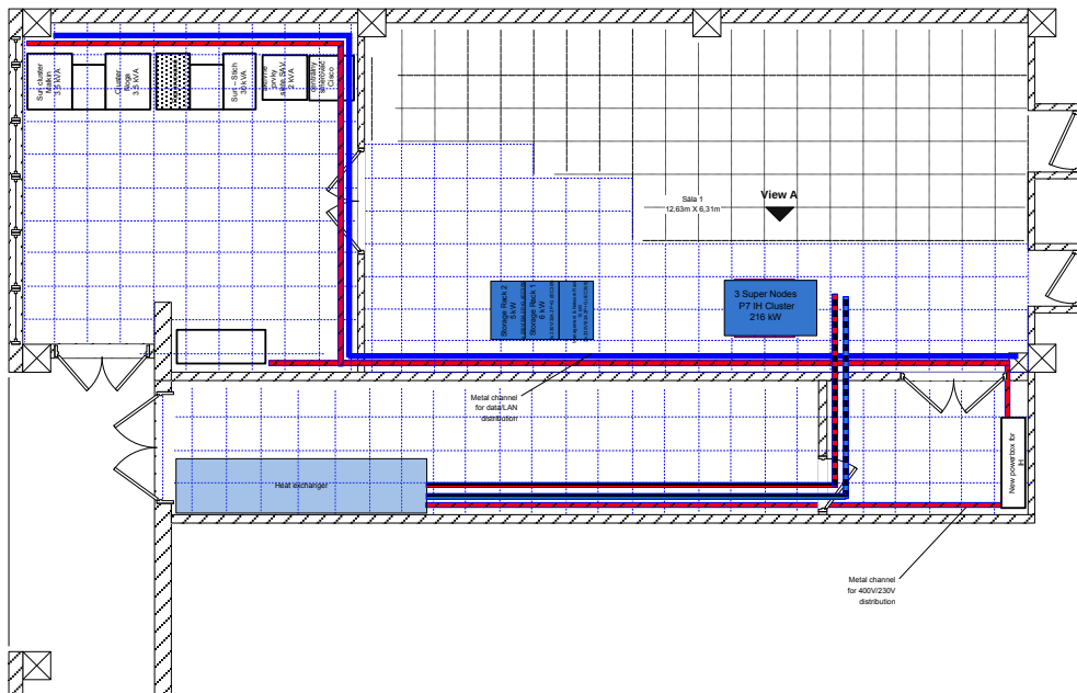
Obr. 5 : Prenesenie zariadení do malej sály a dokončenie podlahy
