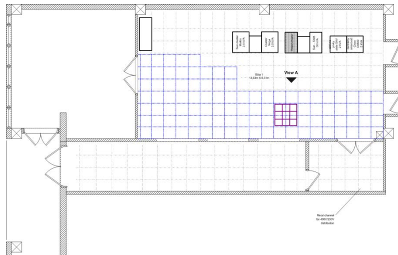
Obr. 3 : Stav rekonštrukcie podlahy vo veľkej sále (modrým osadená nová podlaha)
