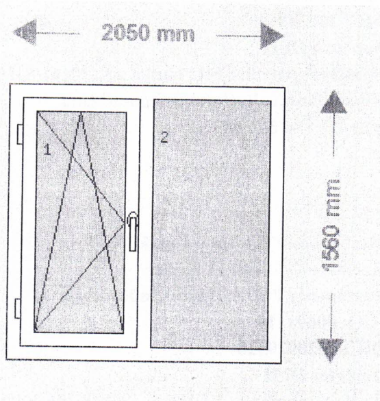
Vnútrotný pohľad
