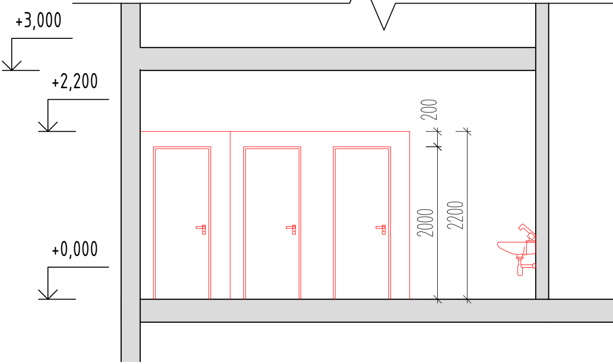
REZ B-B'
