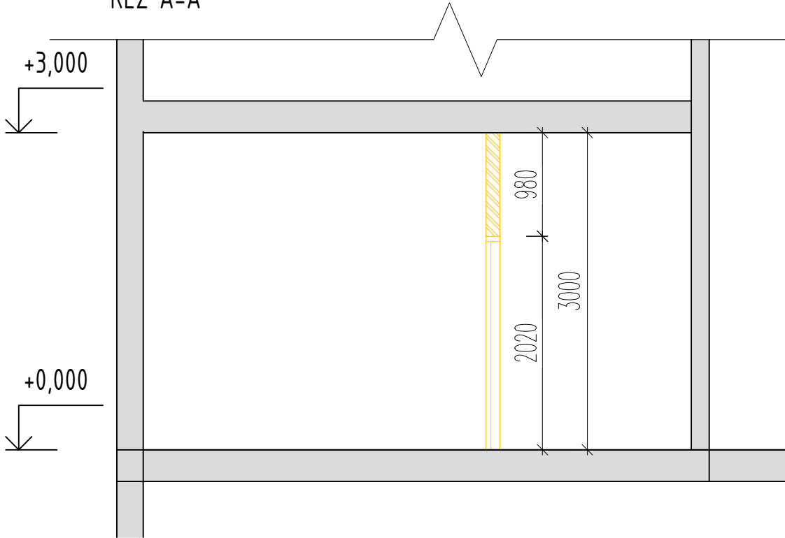
REZ A-A'
