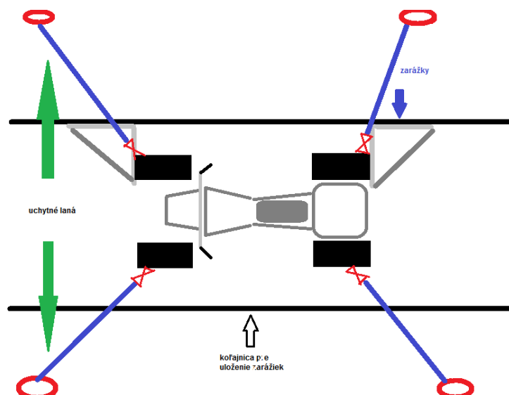
Obr. 5 Upevňovanie štvorkolky
