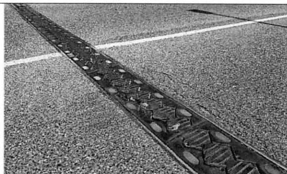
Poškodenia vozovky pred a za DZM
