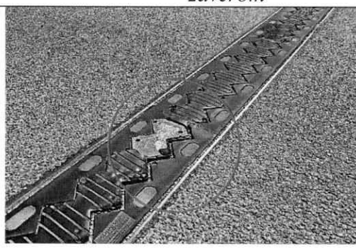
Priečne trhliny s viacnásobným výskytom. Rozpad asfaltového krytu v mieste za mostným záverom
