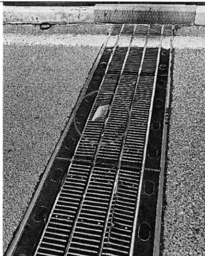
Lokálne odhalené oceľové segmenty gumokovových modulov
