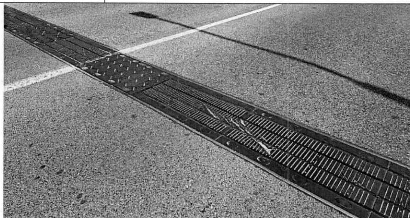
Pohľad na DZM (dĺžka 10m medzi obrubníkmi) – poškodených 10ks gumokovových modulov o rozmeroch 0,55 x 1,0m
