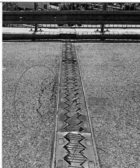
Priečne trhliny s viacnásobným výskytom. Rozpad asfaltového krytu v mieste za mostným záverom
