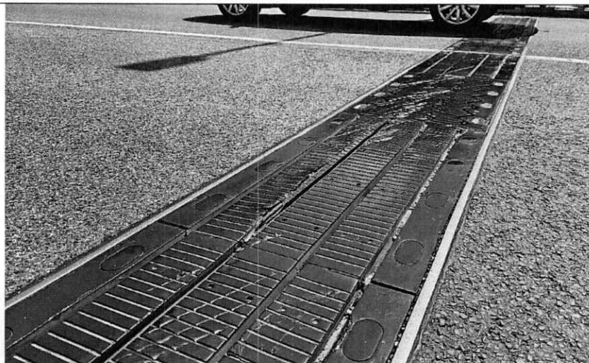
Mechanické poškodenia gumokovových modulov MZ, lokálne porušené kotviace záliveky
