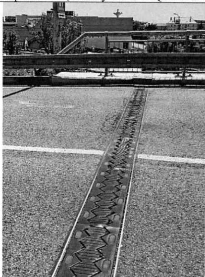
Pohľad na DZM (dĺžka 10m medzi obrubníkmi) – poškodených 10ks gumokovových modulov
