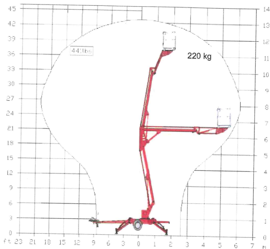
Pracovný diagram pracovnej plošiny EUROPELIFT TM13G
