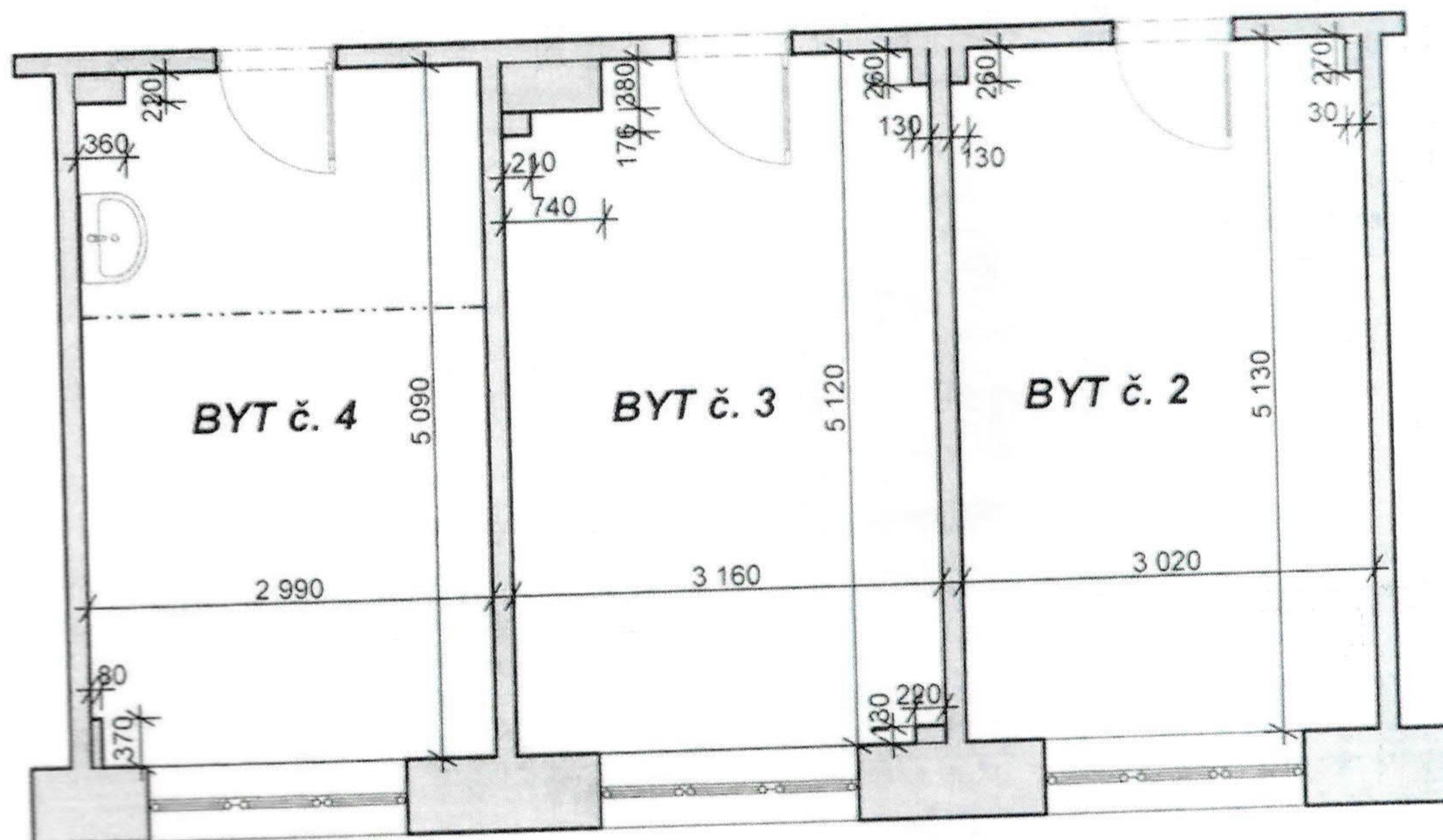
Schematický pôdorys BYTOV č. 2, 3, 4 na 1.podzemnom poschodí
