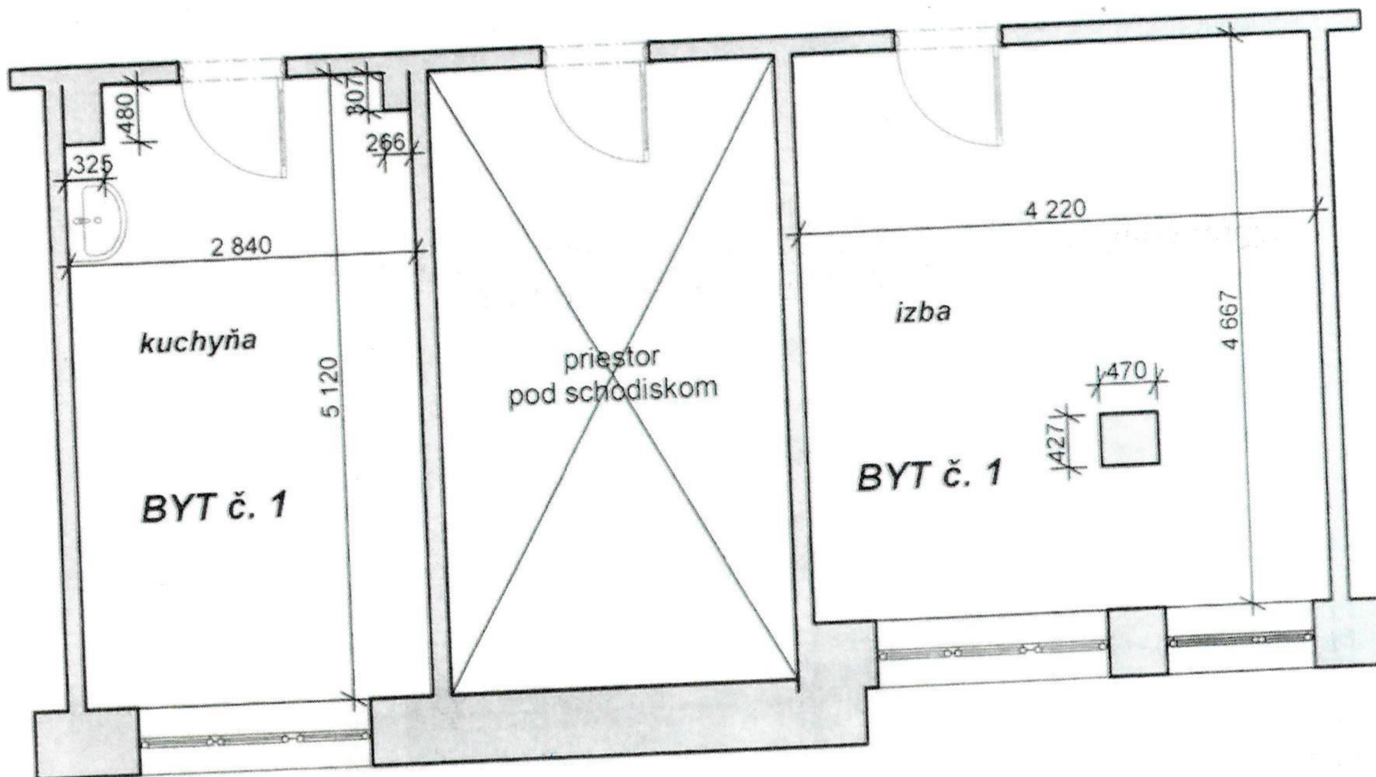
Schematický pôdorys BYTU č. 1 na 1.podzemnom poschodí
