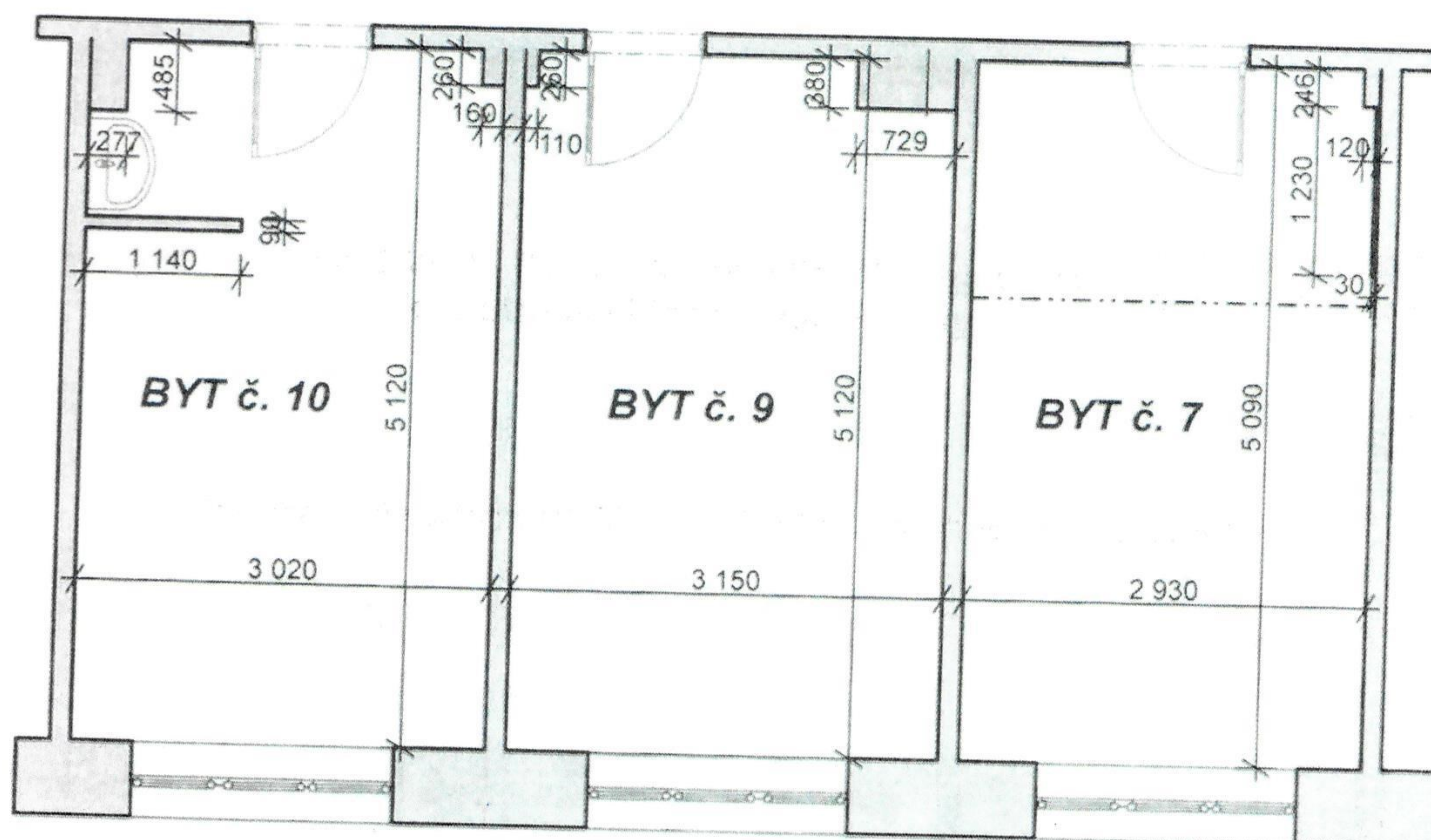
Schematický pôdorys BYTOV č. 7, 9, 10 na 1.podzemnom poschodí
