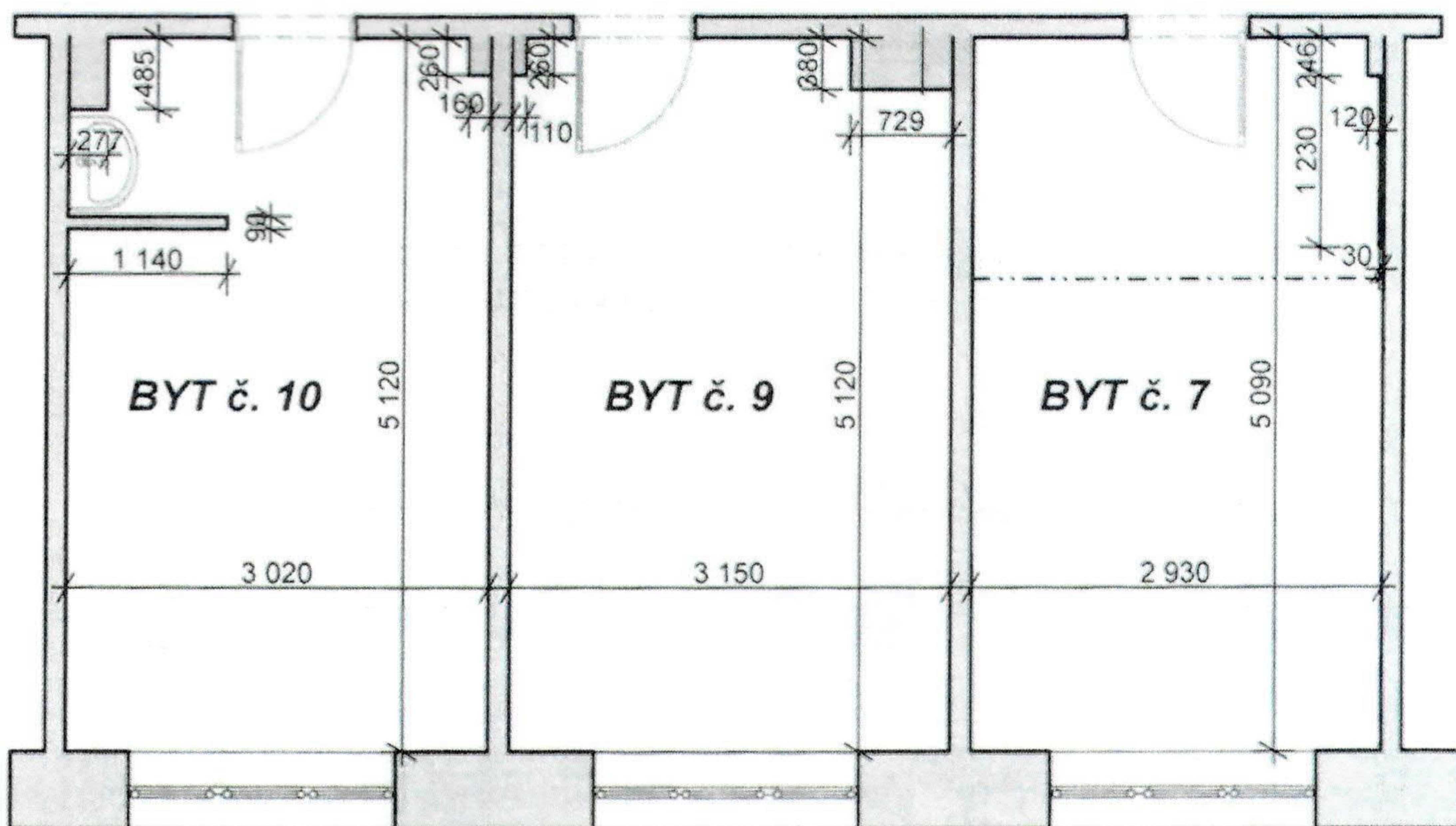
Schematický pôdorys BYTOV č. 7, 9, 10 na 1.podzemnom poschodí
