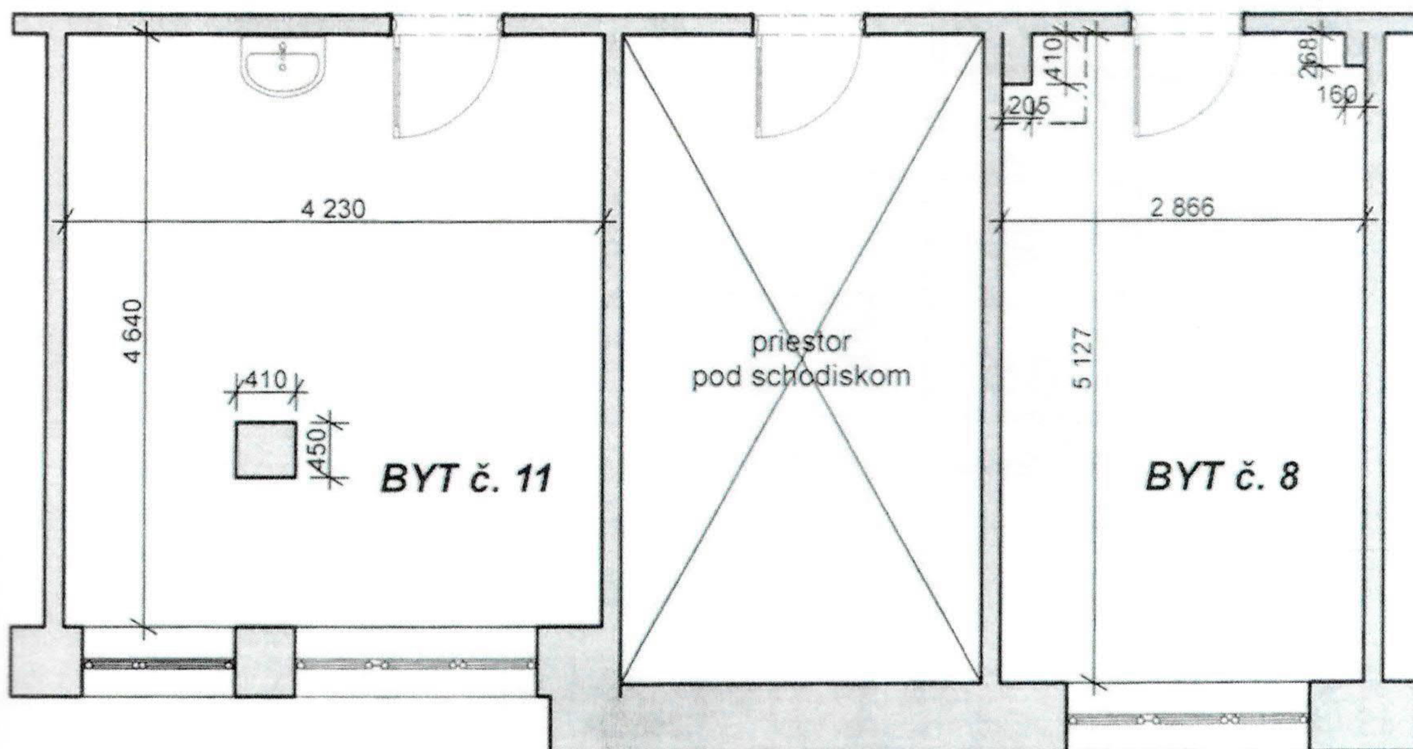
Schematický pôdorys BYTOV č. 8 a 11 na 1.podzemnom poschodí
