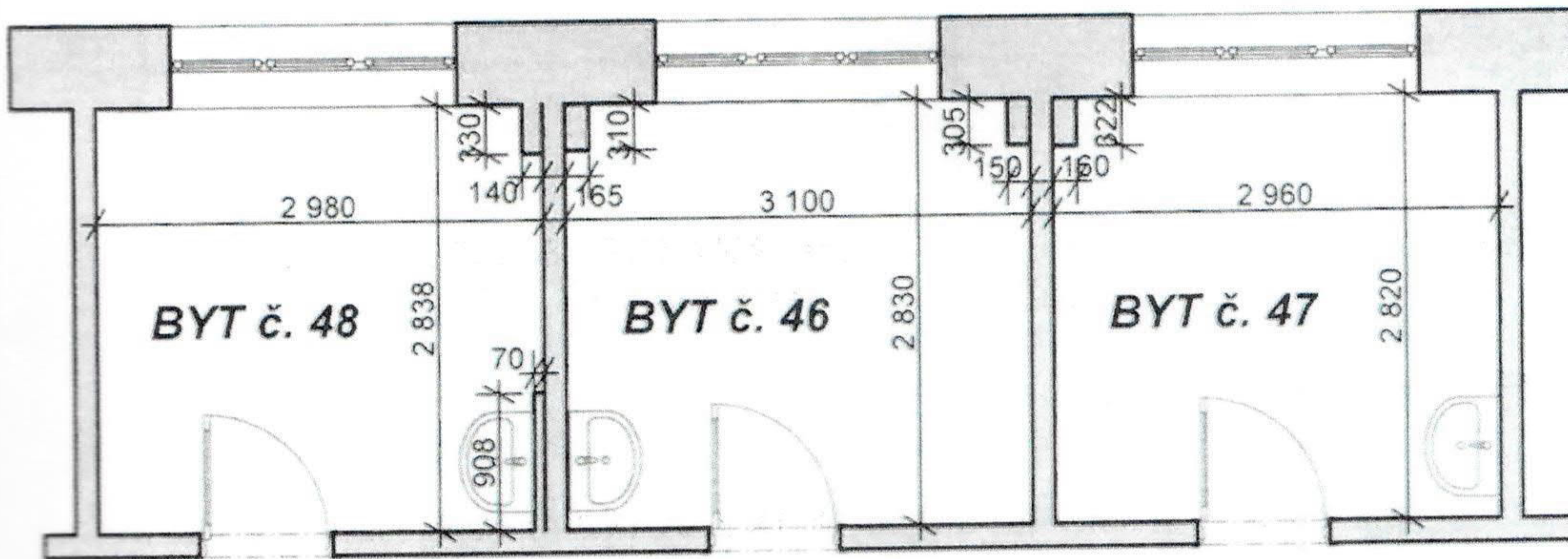
Schematický pôdorys BYTOV č. 48, 46 a 47 na 3.nadzemnom poschodí
