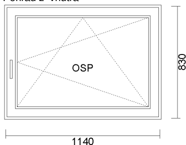
3) OKNO PVC (OSP). 1140x830 Pohľad z vnútra
