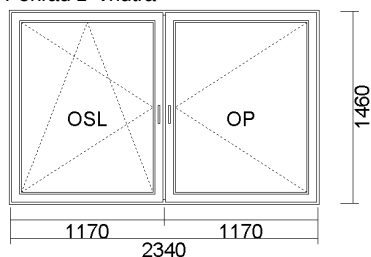
7) OKNO PVC (OSL+OP). 2340x1460 Pohľad z vnútra
