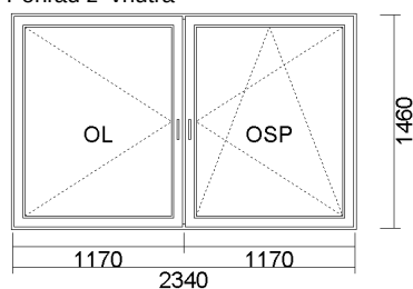
5) OKNO PVC (OL+OSP). 2340x1460 Pohľad z vnútra
