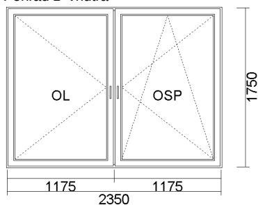
8) OKNO PVC (OL+OSP). 2350x1750 Pohľad z vnútra
