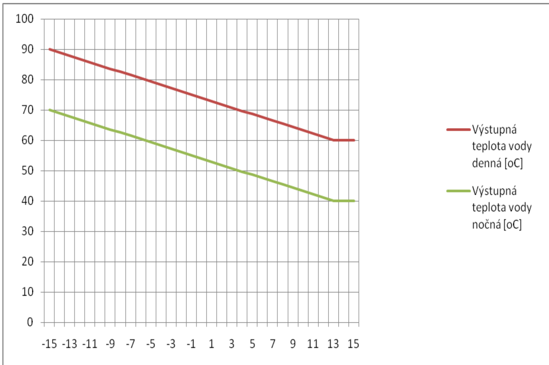
Vykurovací krivka
