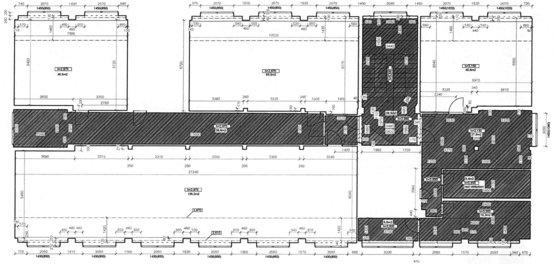
pôdorys 7NP
