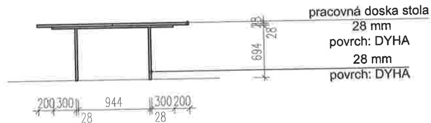
REZ B-B
