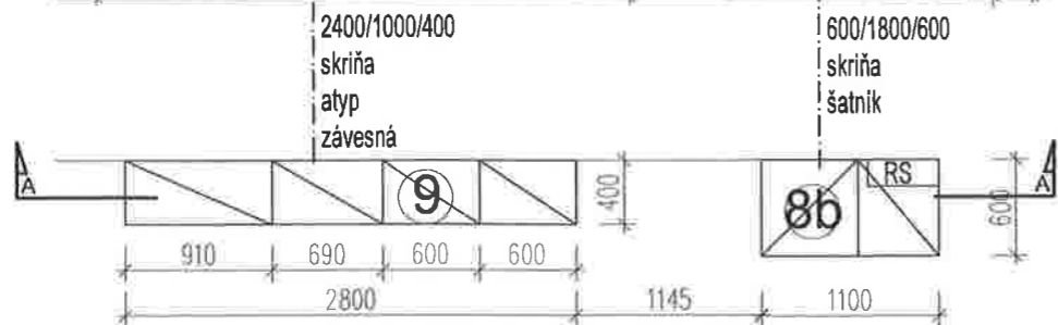
PODORYS
