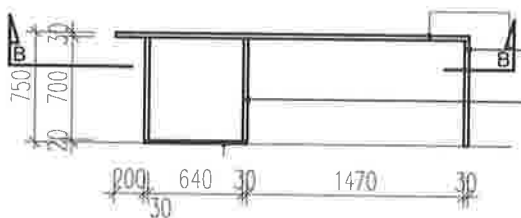
REZ A-A
