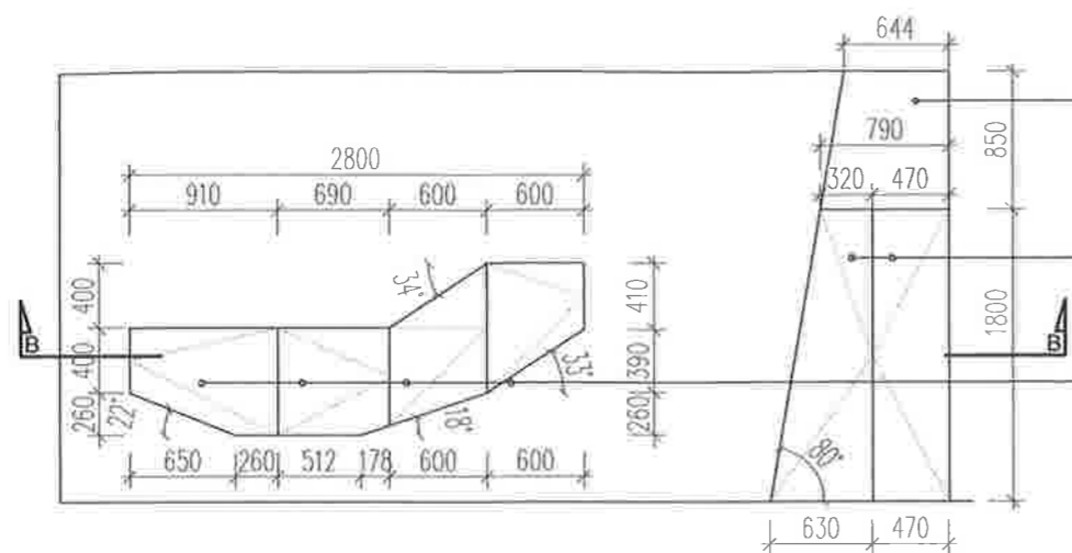
POHLAD 1
