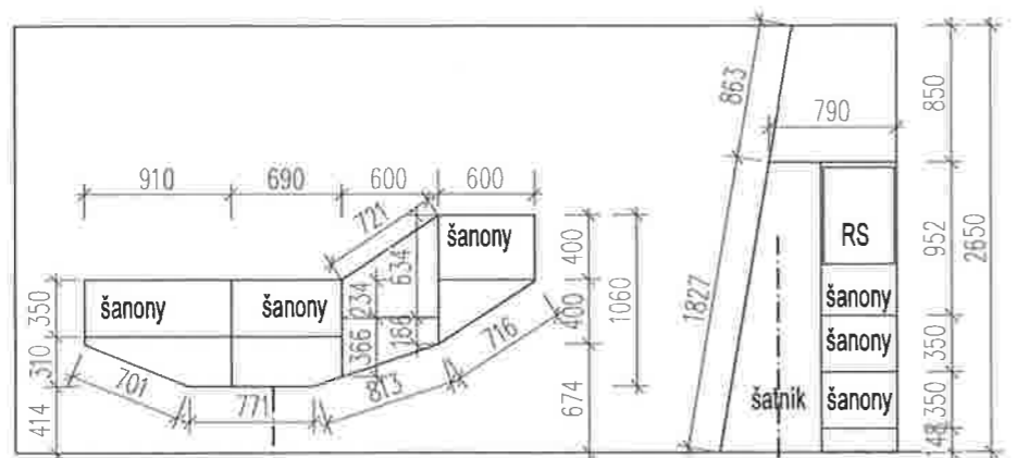
POHLAD 2
