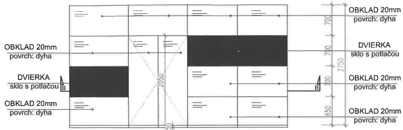
POHLAD 1
