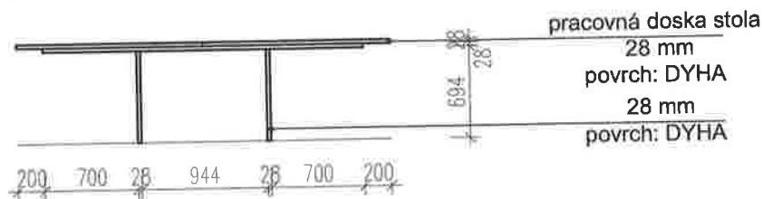
REZ A-A
