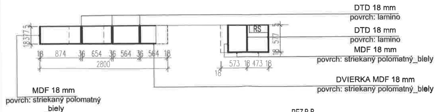
REZ-B-B
