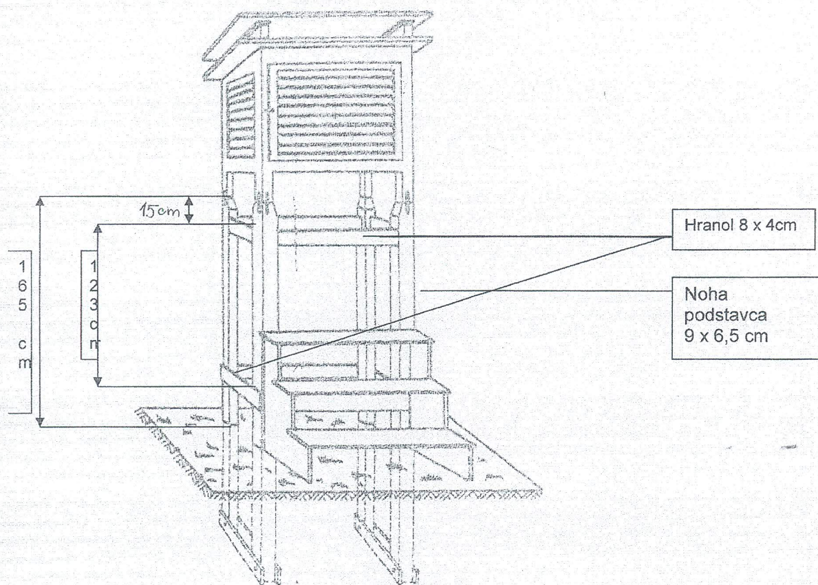
Obr. 4. Velká žaluziové meteorologická bouda
