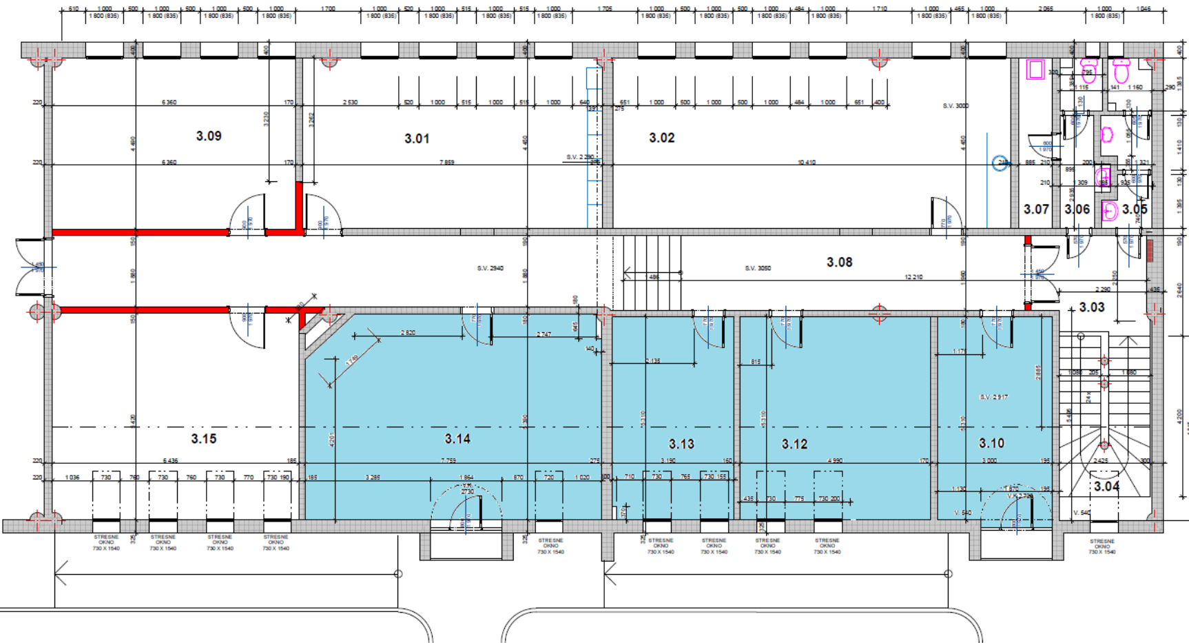
PODORYS 3NP M=1:50
